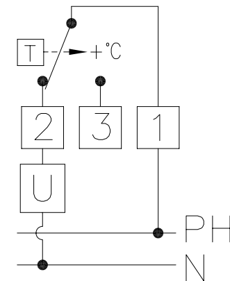
SCHEMA ELETTRICO
